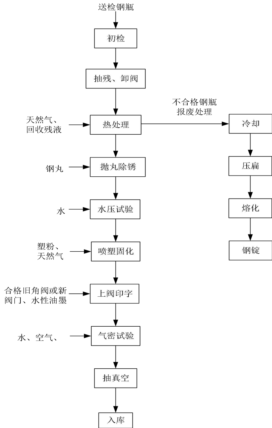
图2 钢瓶检验工艺流程图
