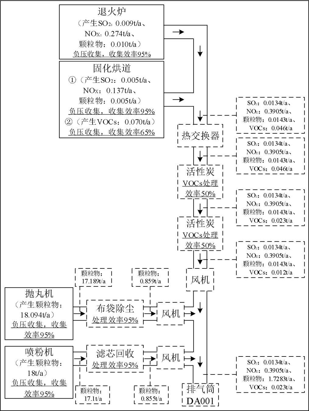
图3 废气走向收集图
