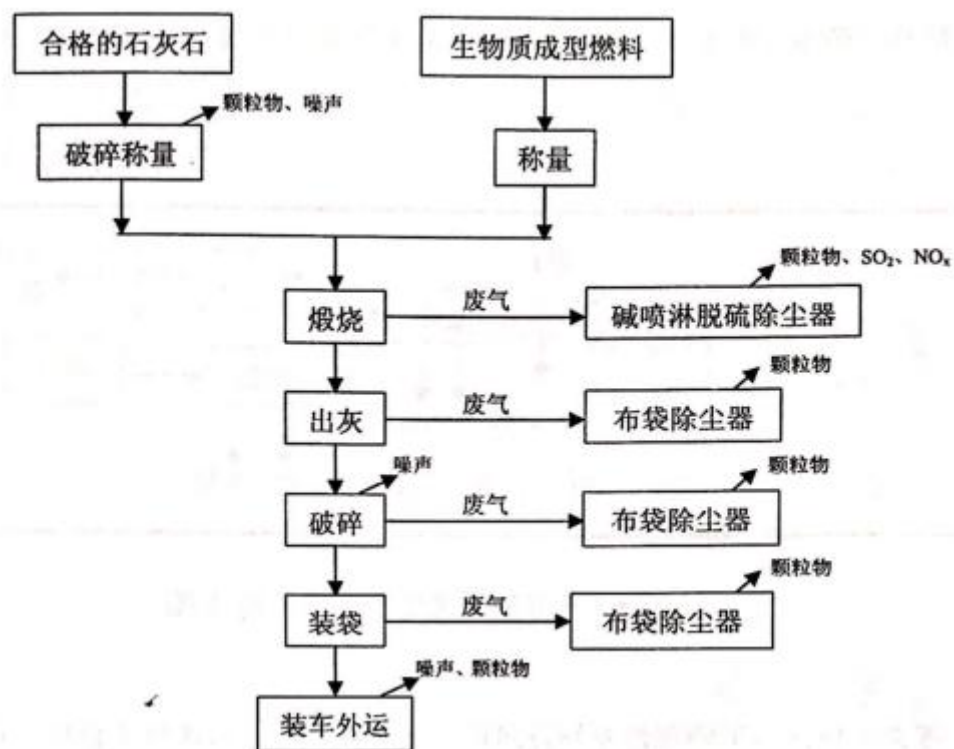
图 1-5 石灰生产工艺流程图
