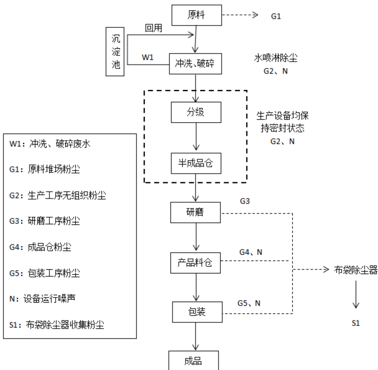
图 5-1 运营期工艺流程及产污环节图
